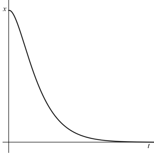
চিত্র ৪: \omega_0 = \gamma হলে বস্তুকণার অবস্থান বনাম সময় গ্রাফ
